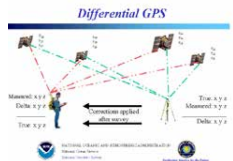
Σχέδιο 5. Λειτουργία του DGPS
