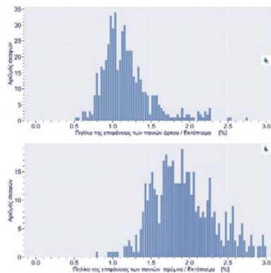
Εικόνα 6: Πηλίκο της επιφάνειας των πανιών όρτσα και πρύμα δια του εκποτίσματος
